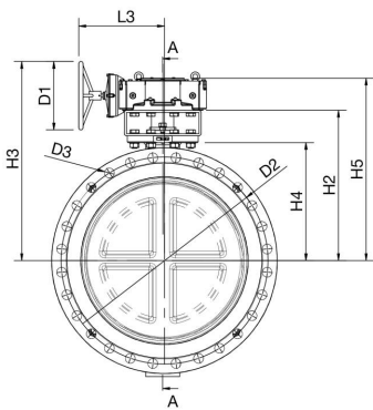
DN 900-1000
