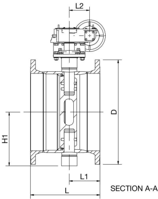
DN 900-1000
