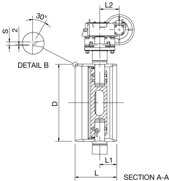
DN 900-1200
