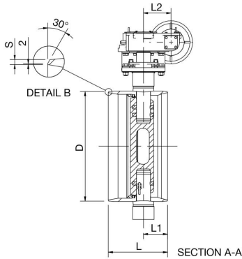
DN 900-1200
