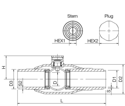
DN 20-125
